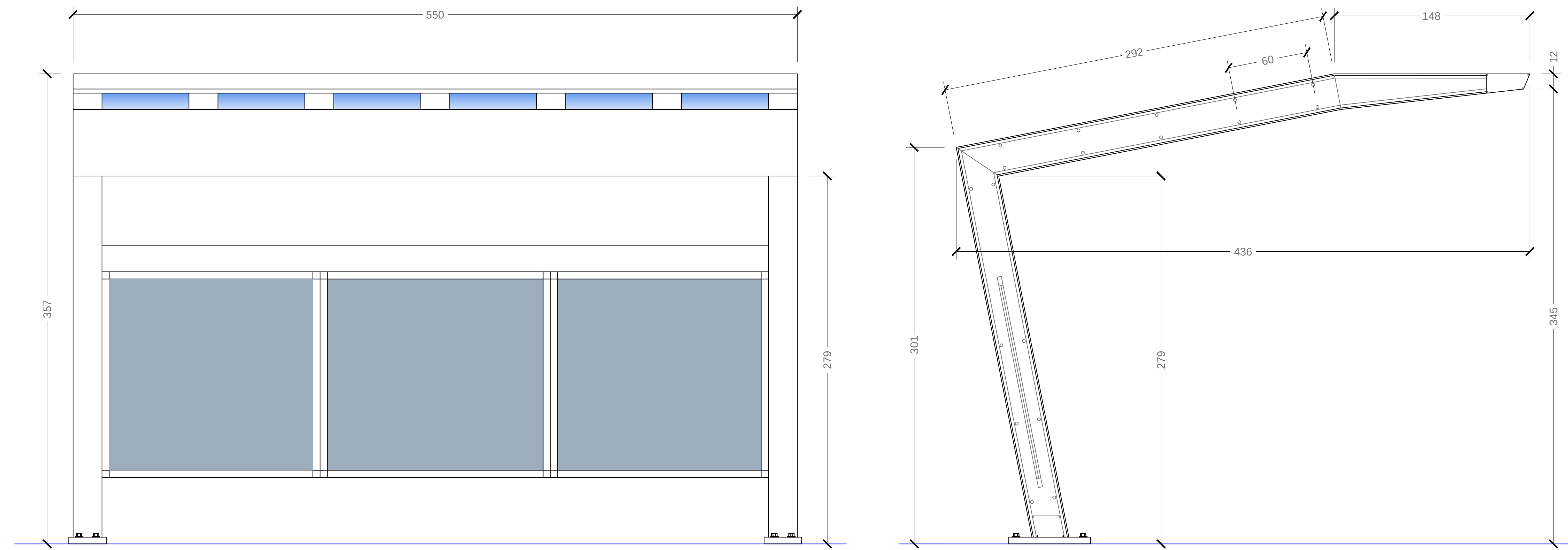
Pensiline Scala 1:20
