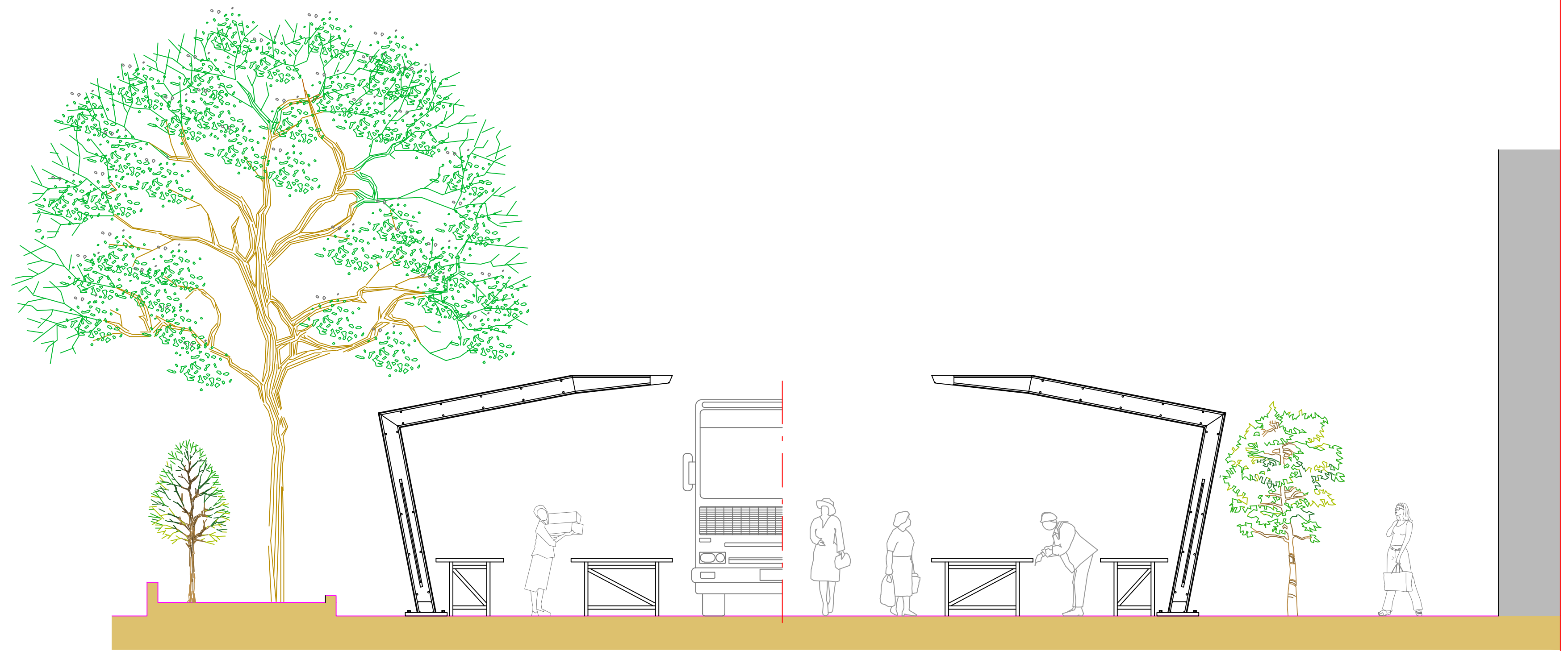
SEZIONE A-A Scala 1:50
